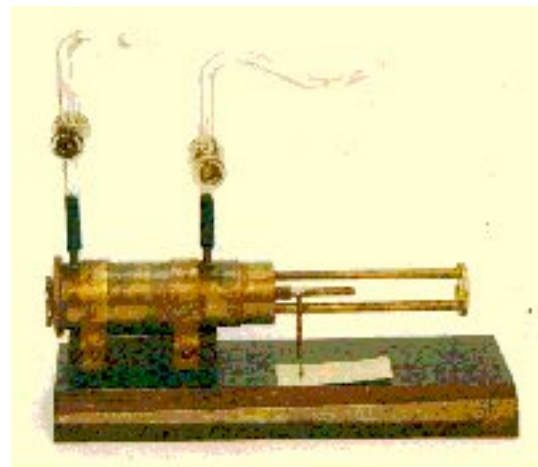
Chambre de désintégration nucléaire, Rutherford
